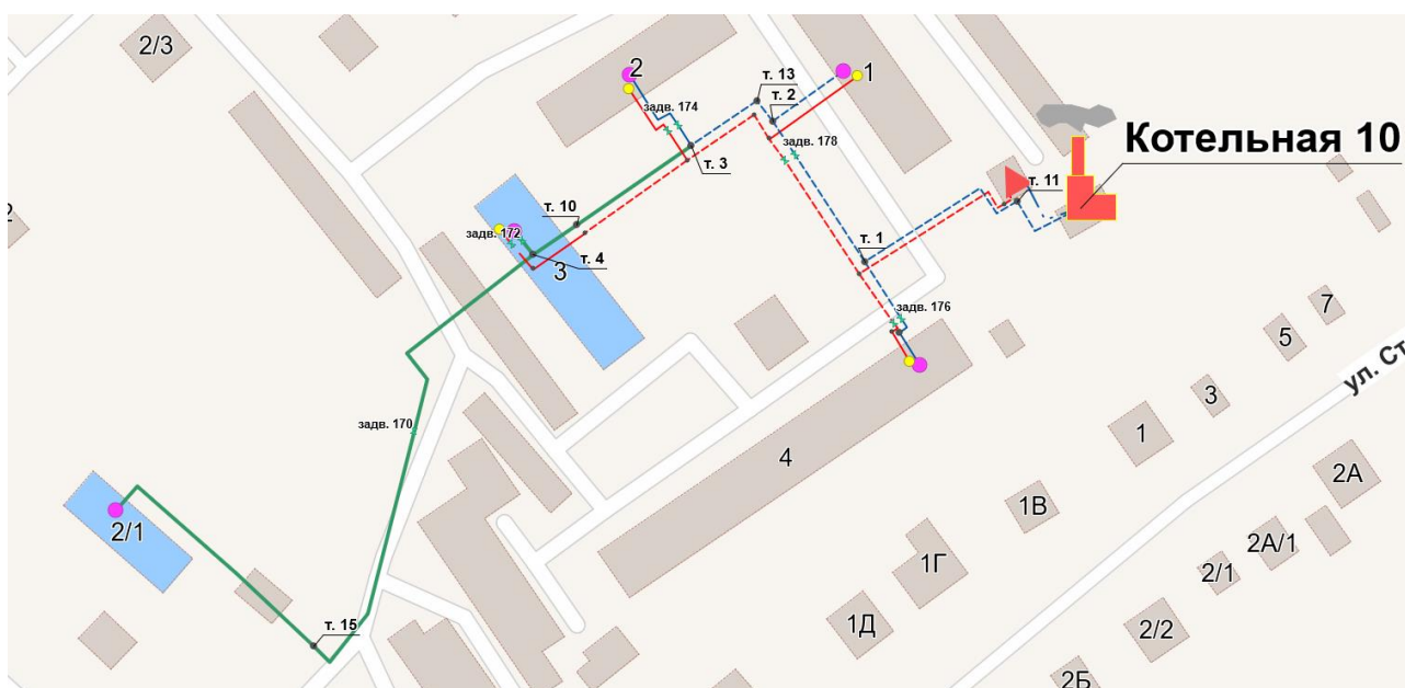
Рисунок 14 Визуализация отключения запорной арматуры на котельной №10 г. Темрюк, Набережная, 5к
