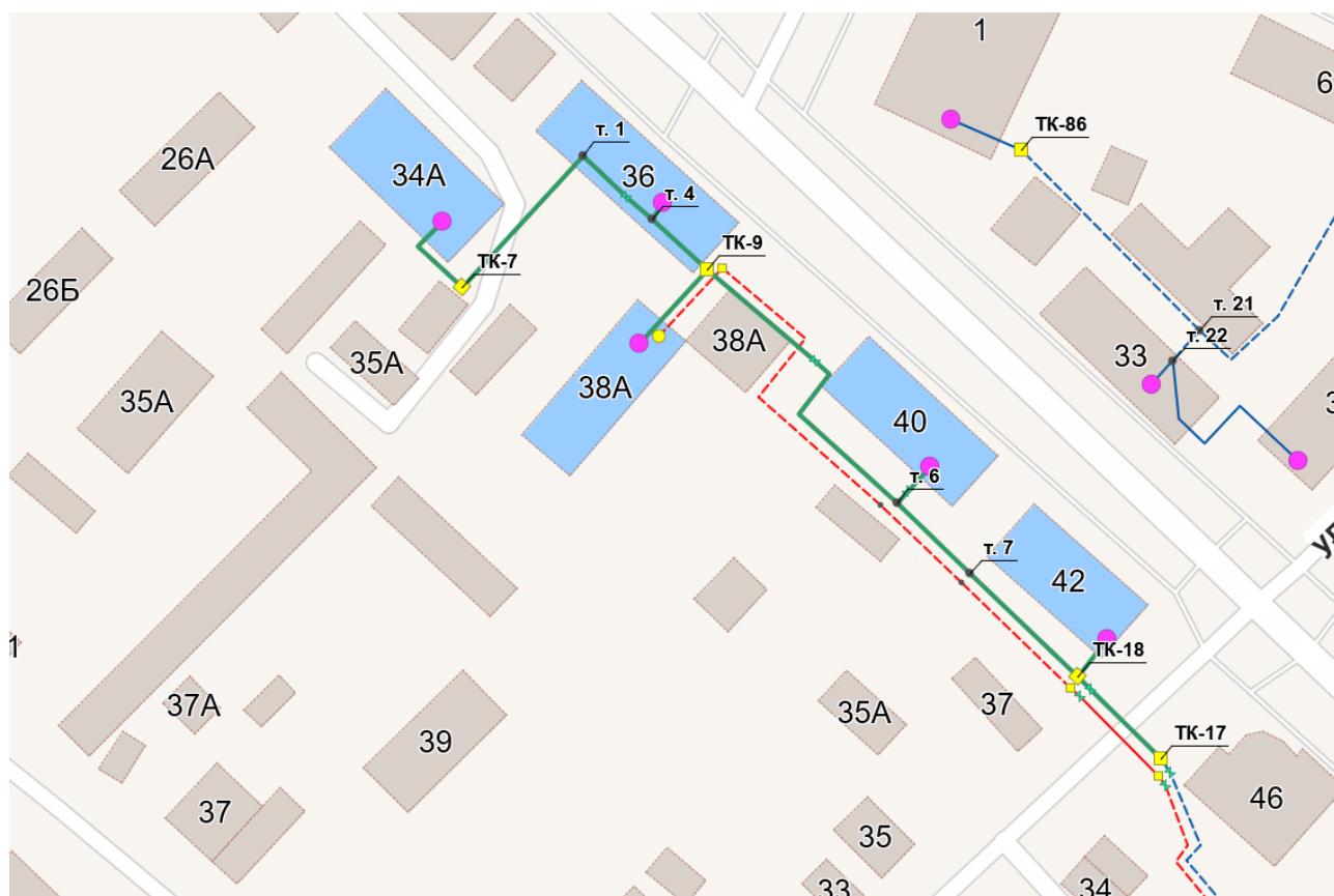
Рисунок 6. Визуализация отключения запорной арматуры на котельной №1 г. Темрюк, Ленина, 63а
